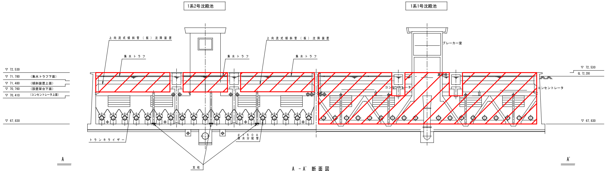
A - A' 断面図
