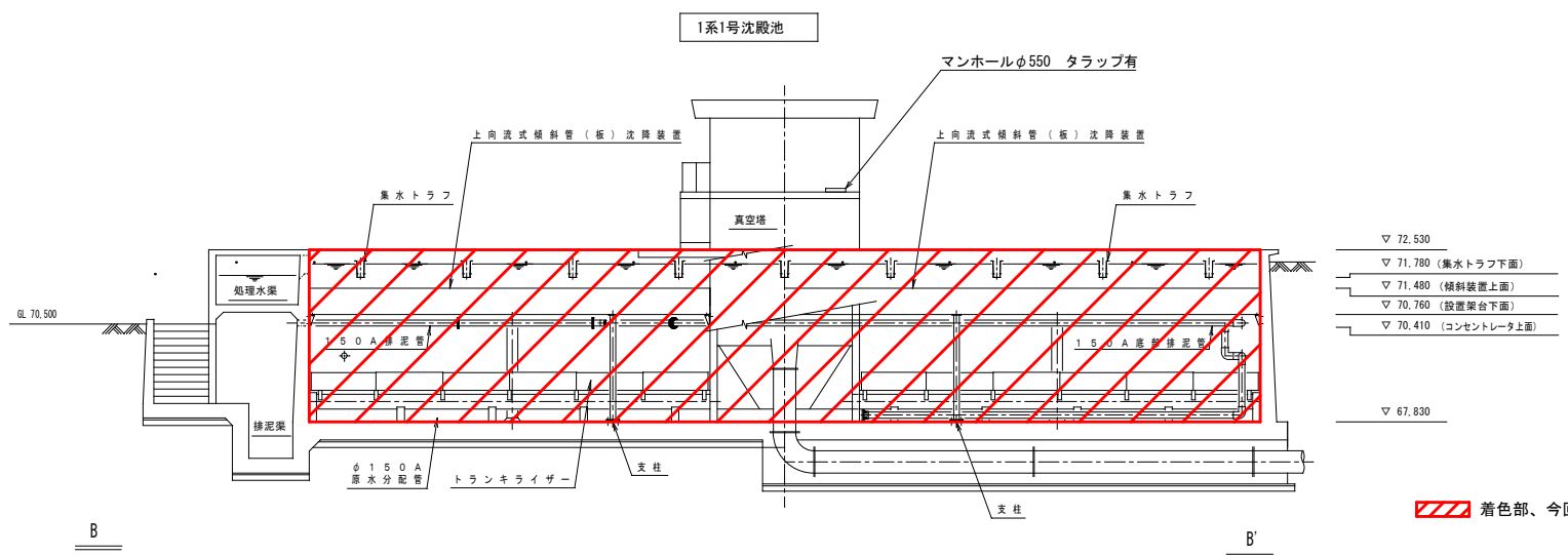
B - B' 断面図
