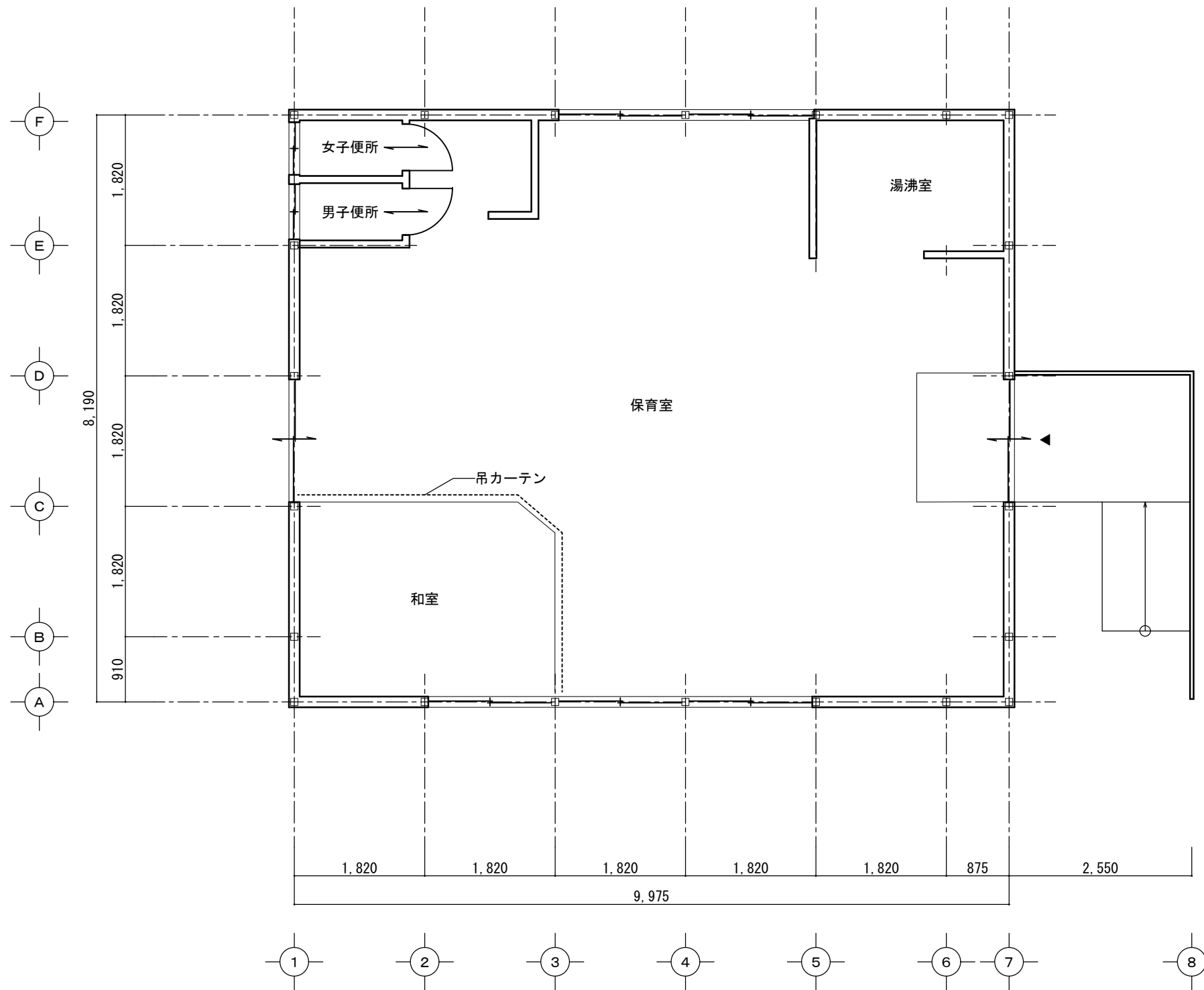
平面図 1/50
