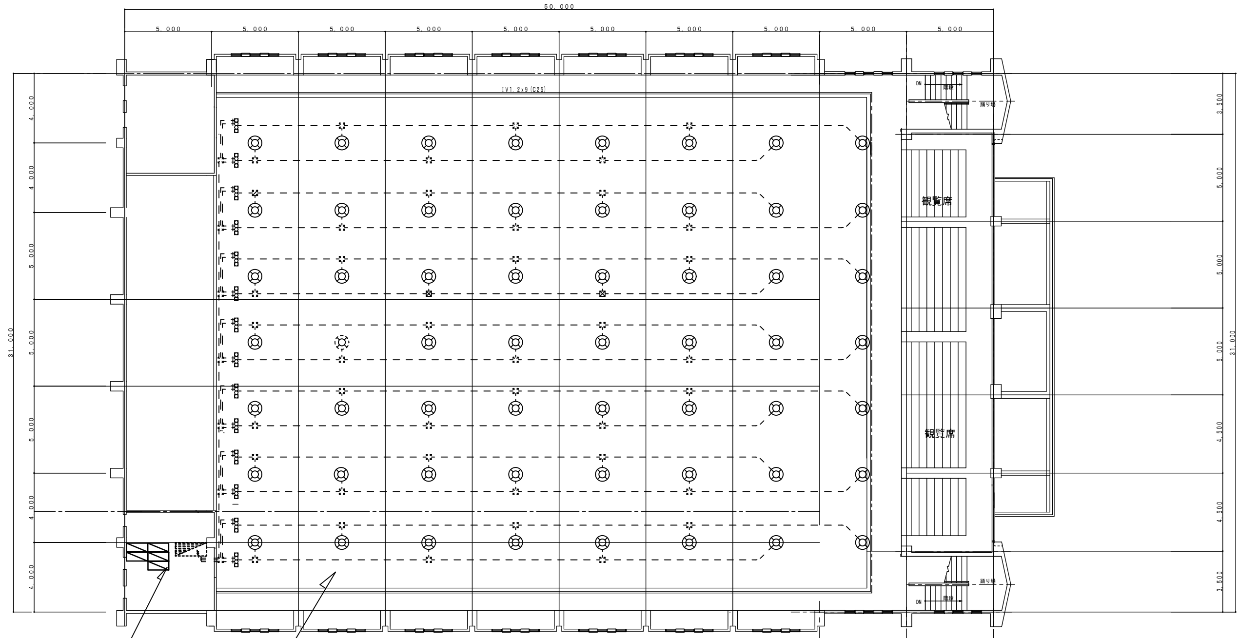
2階上部平面図
