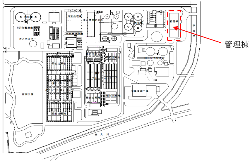
図1-2 中央浄化センター管理棟1階 *電源は配置位置まで延長コードにて設置
