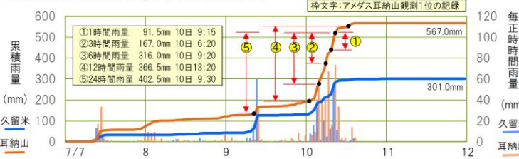
累積雨量・時間雨量図(アメダス久留米・耳納山)
