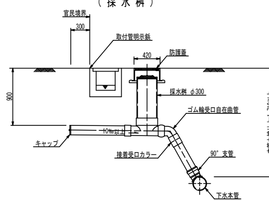
取付管掘削標準断面図 S=1:30
