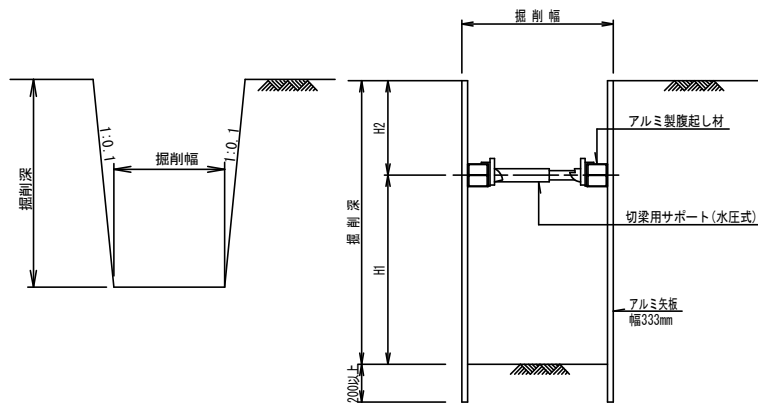
断面図①
