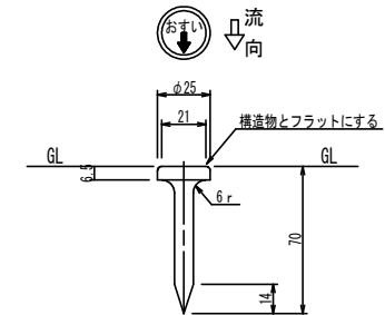
取付管位置明示板設置図 S=1:2
