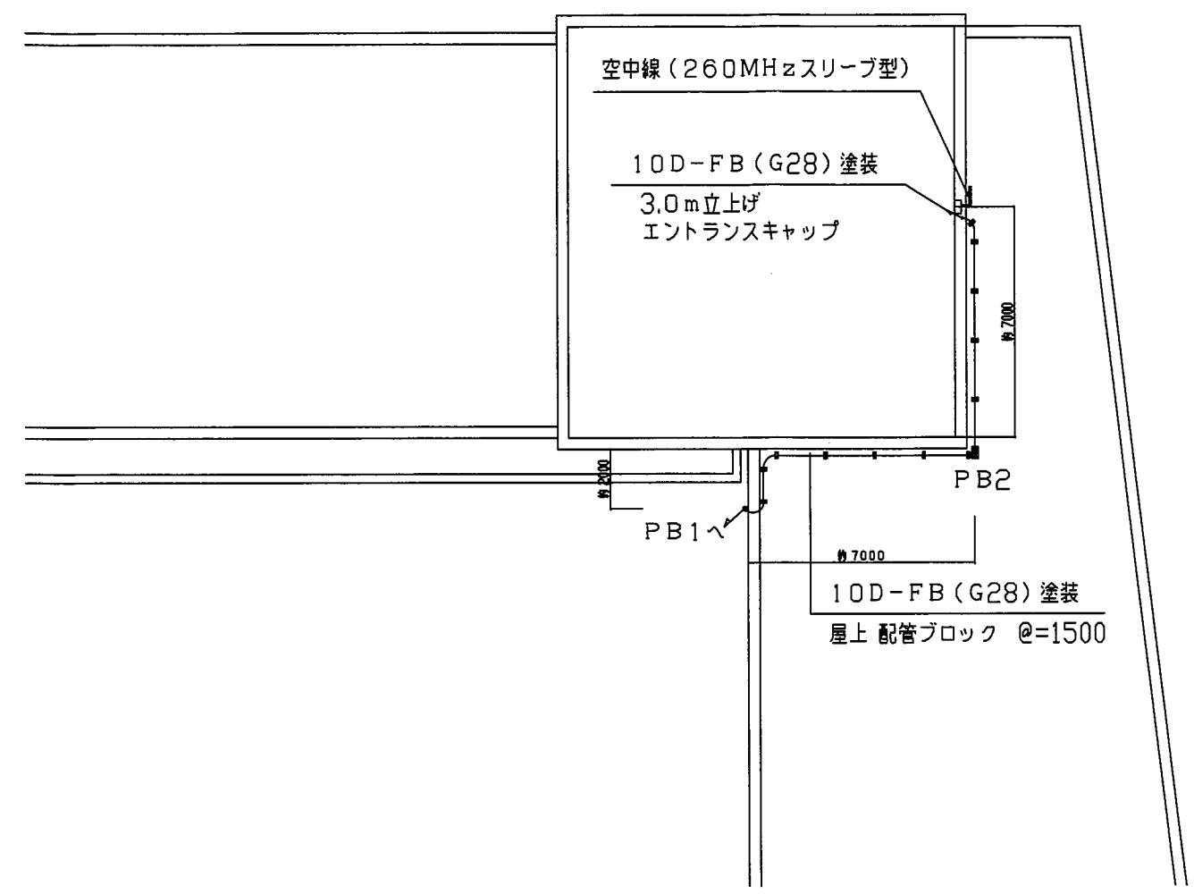
R階 詳細平面図
