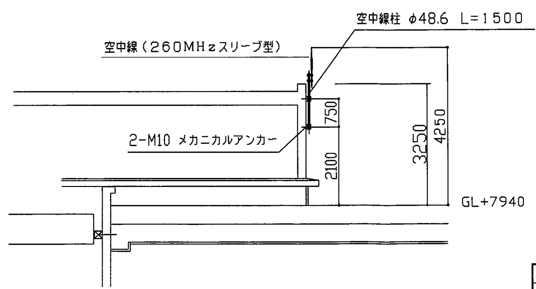
空中線取付図
