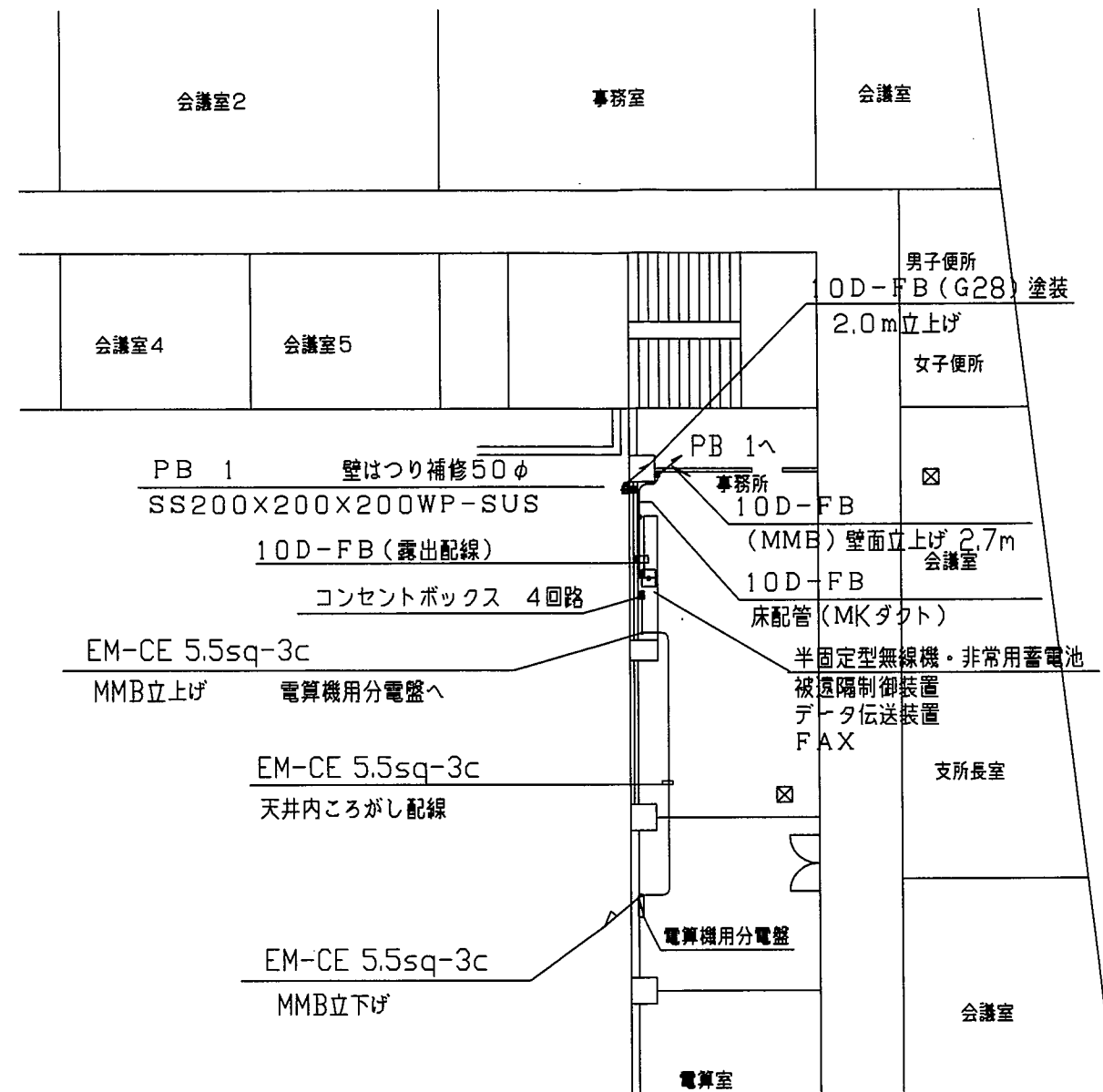
2階 詳細平面図
