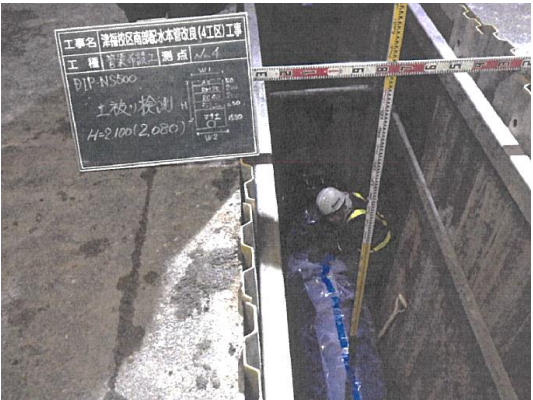
施工状況
