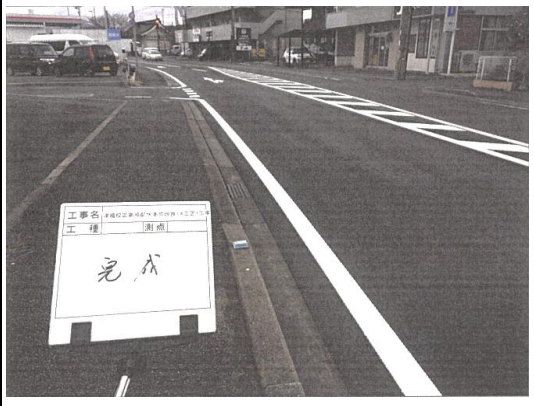
竣工
