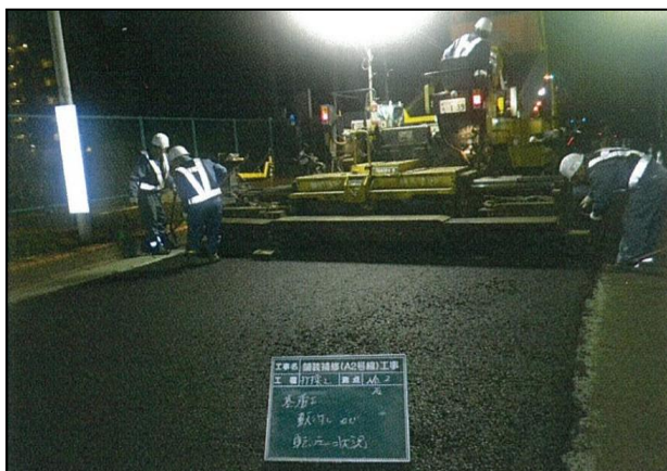
施工状況
