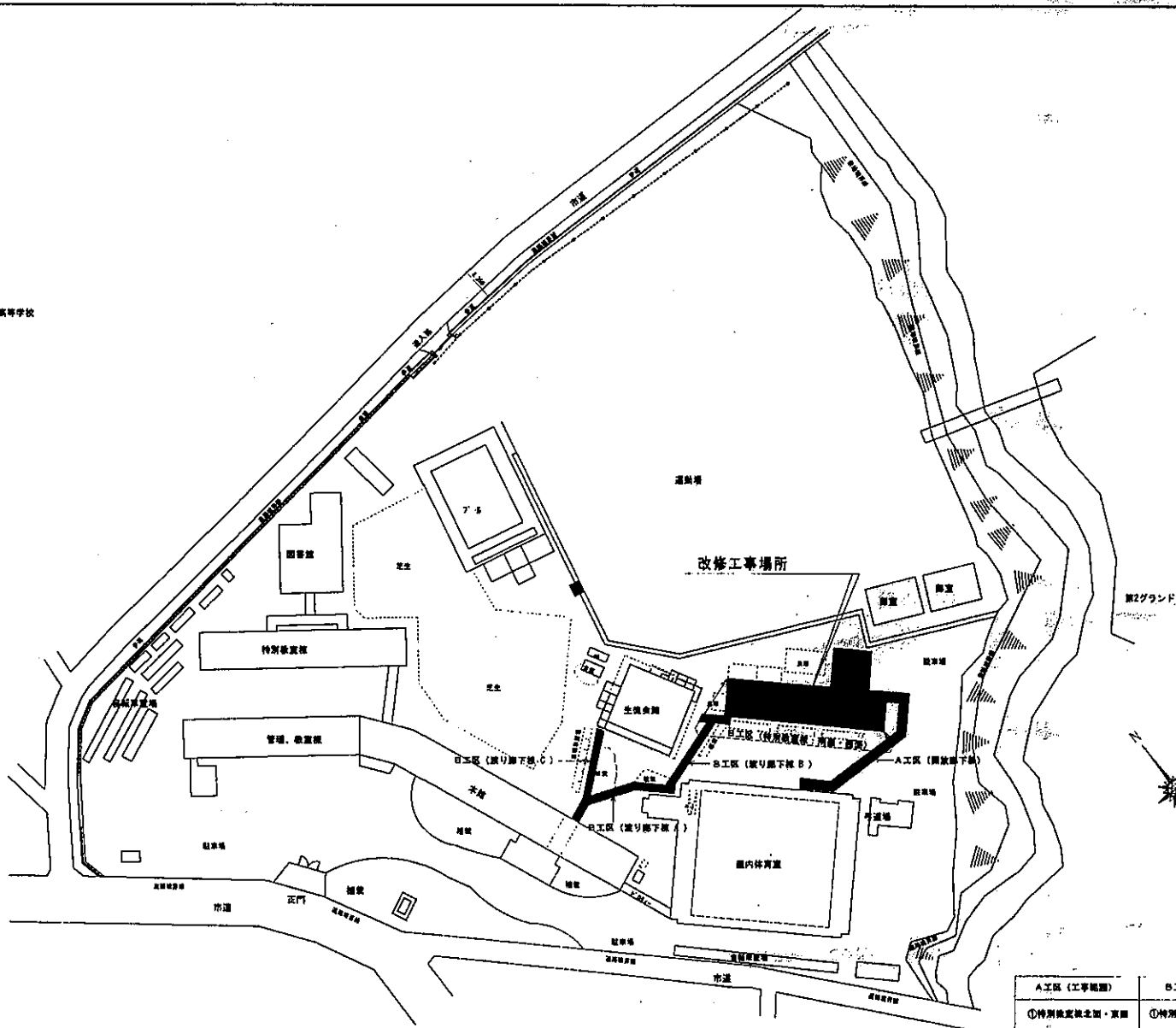
配置図 S=1/800
