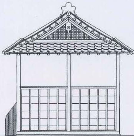
東立面図
