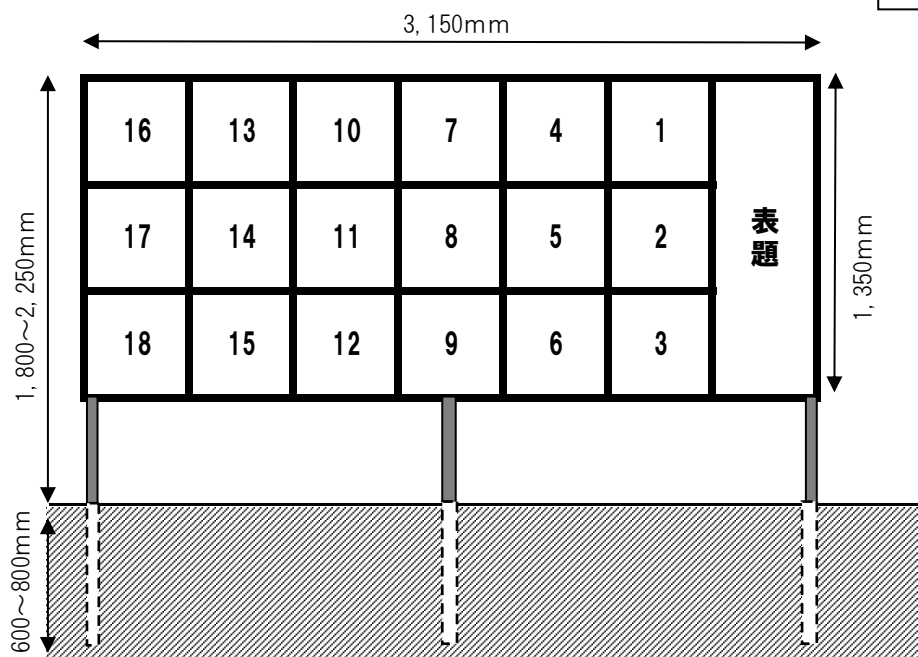
正面図
