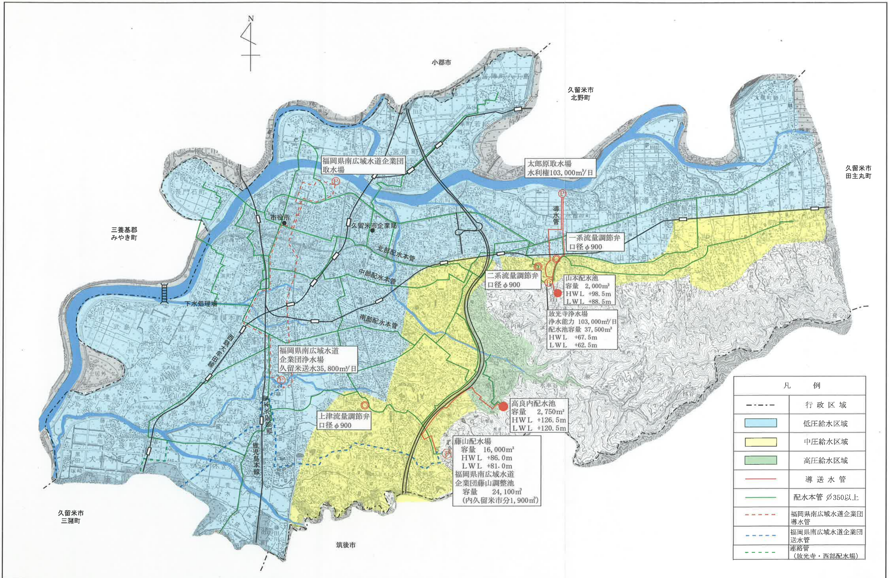
給水区域図その1 (放光寺浄水場系、藤山配水場系)
