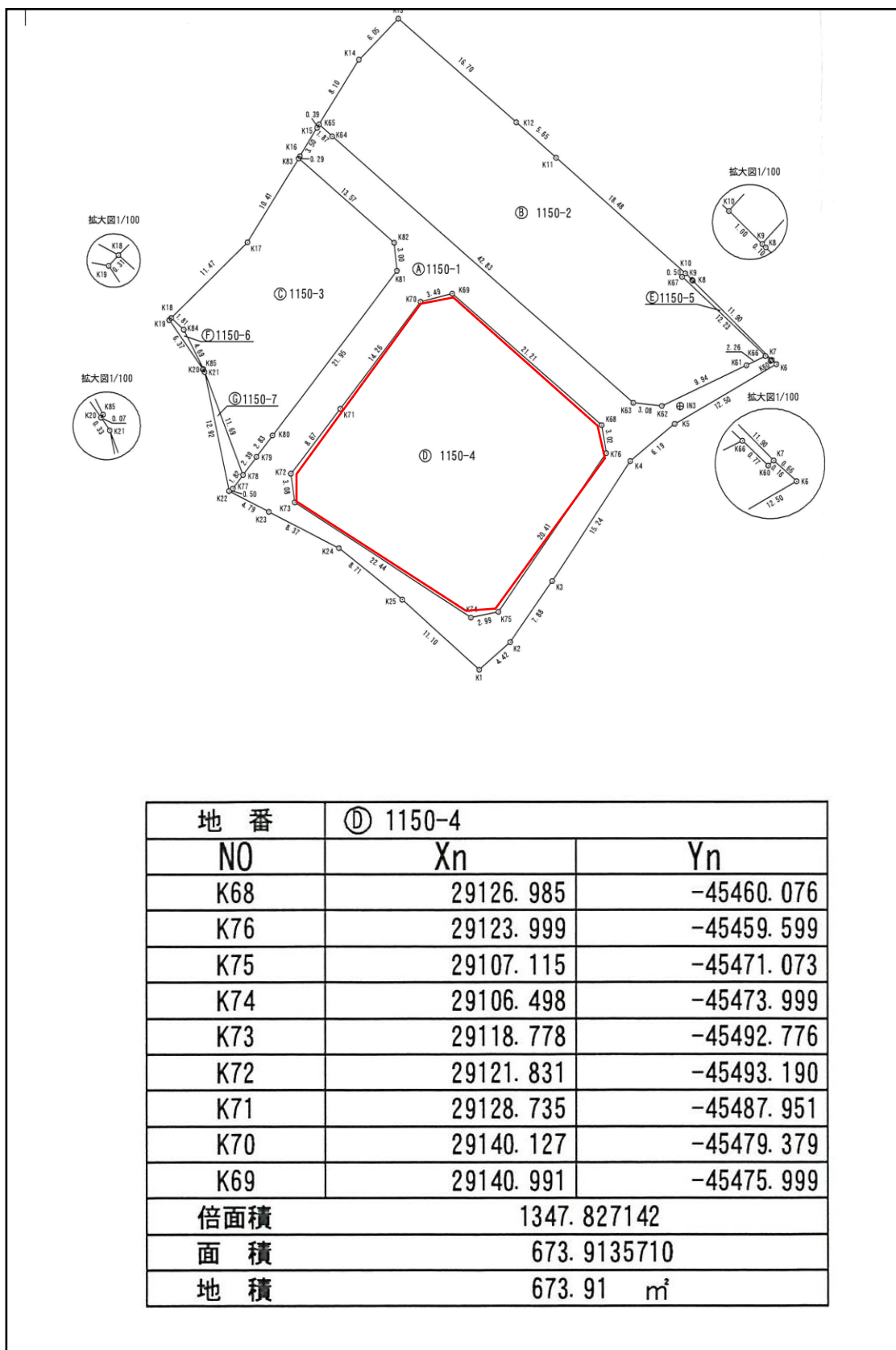
平面图
