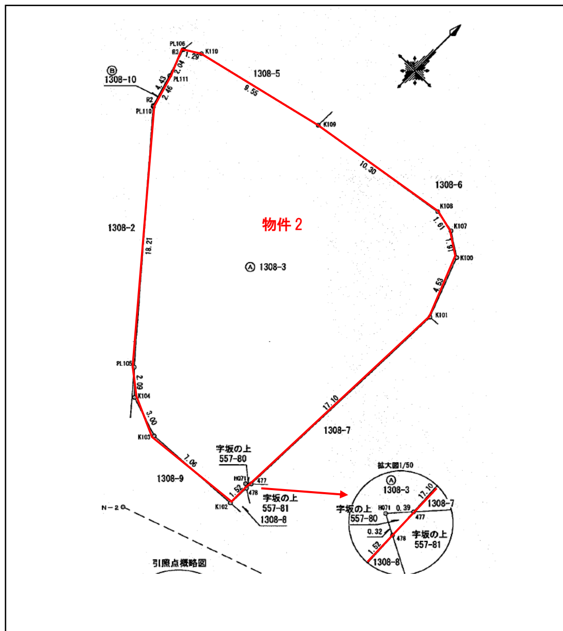
平面図
