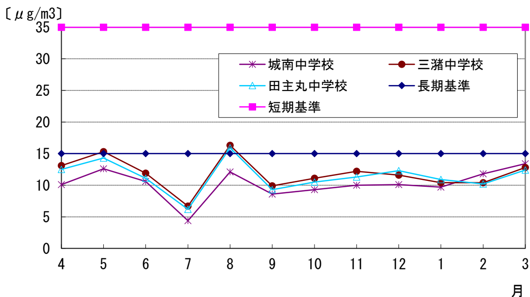
図2-1-10 令和2年度 PM2.5濃度 年間変化(月平均値)
