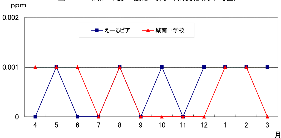
図2-1-2 令和2年度 二酸化いおう 年間変化(月平均値)
