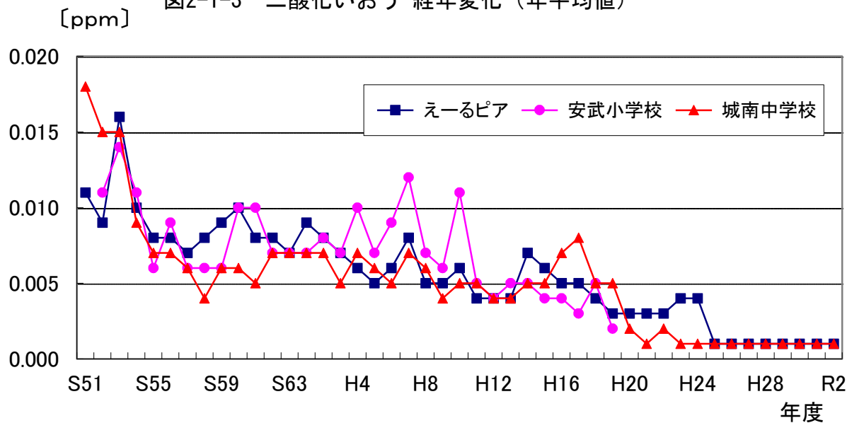
図2-1-3 二酸化いおう 経年変化 (年平均値)
