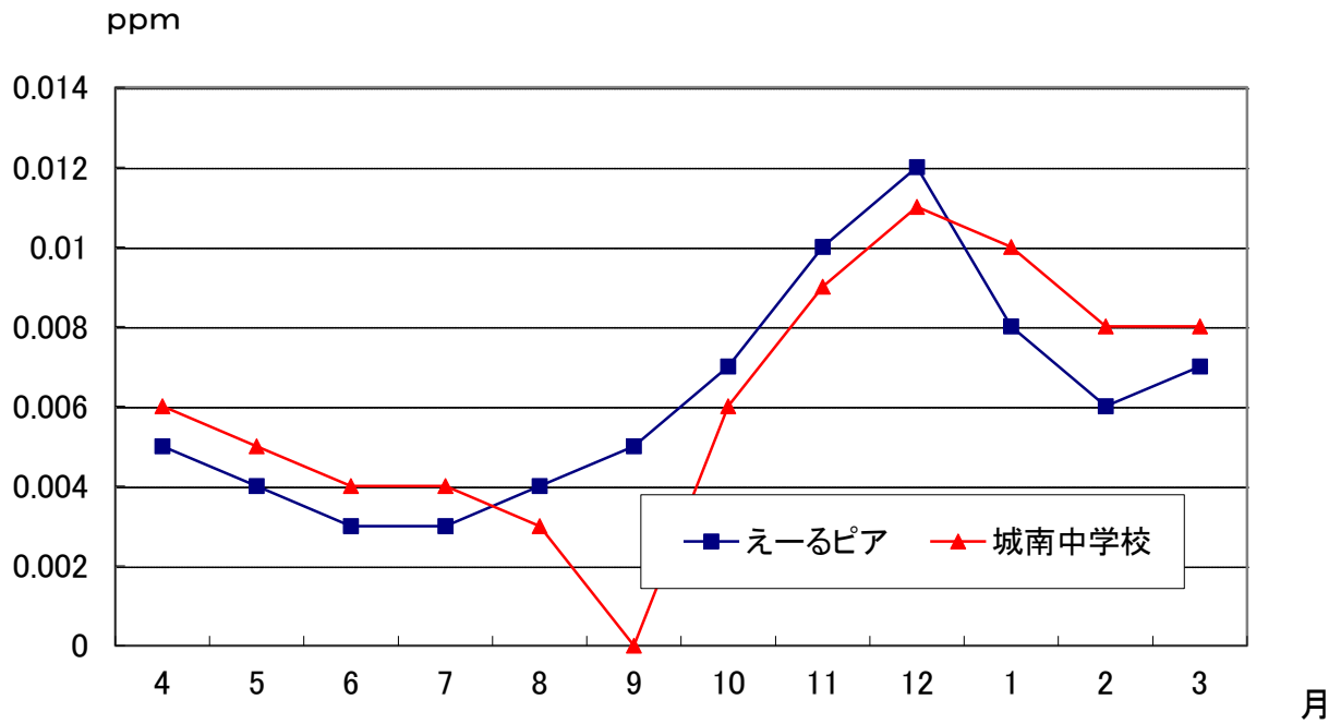
図2-1-6 令和2年度 二酸化窒素 年間変化(月平均値)
