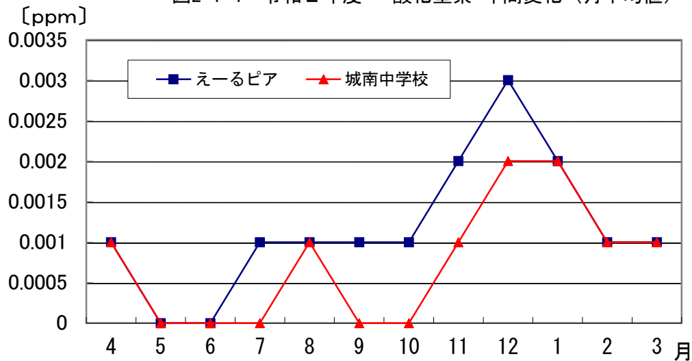
図2-1-4 令和2年度 一酸化窒素 年間変化（月平均値）
