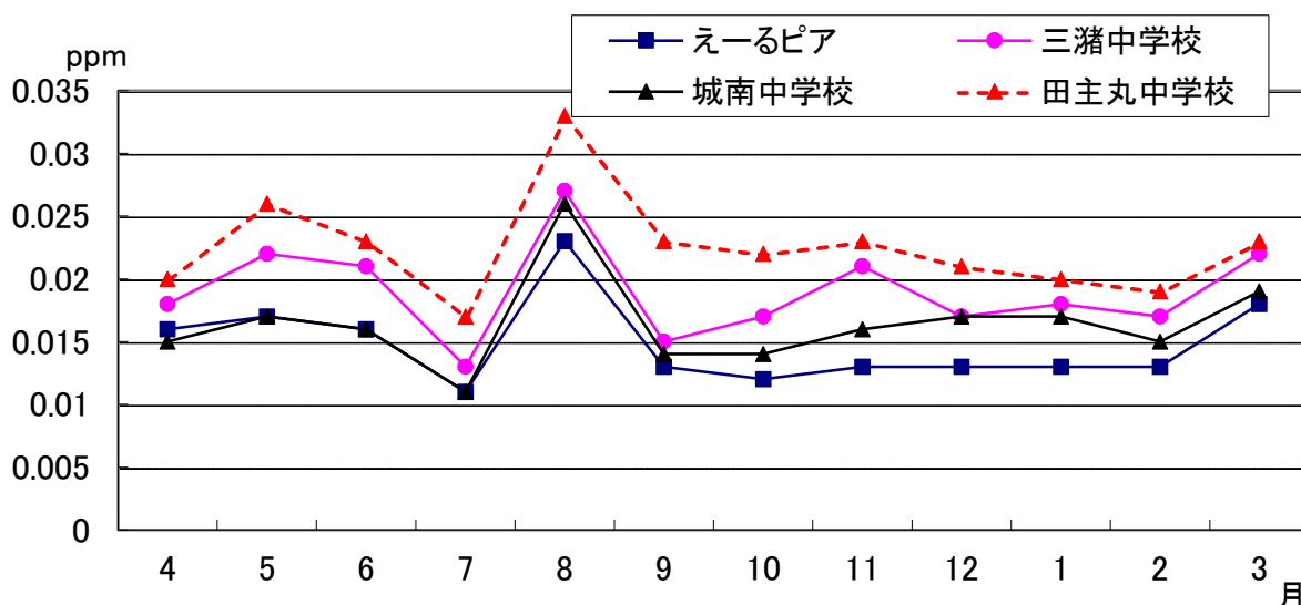
図2-1-8 令和2年度 浮遊粒子状物質 年間変化
