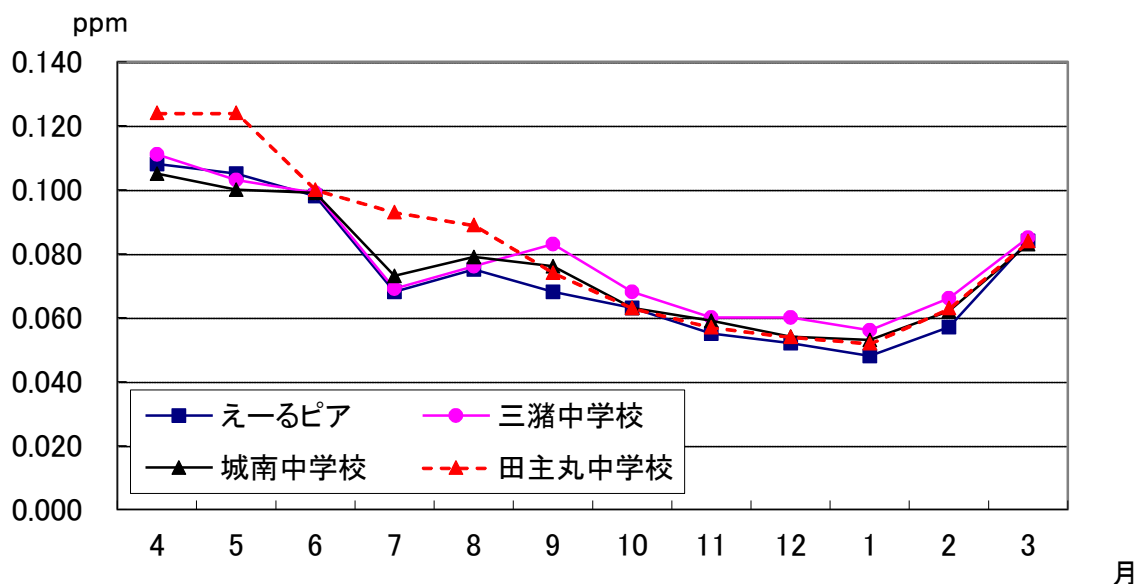
図2-1-12 平成29年度 光化学オキシダント年間変化 （昼間の1時間値の最高値）
