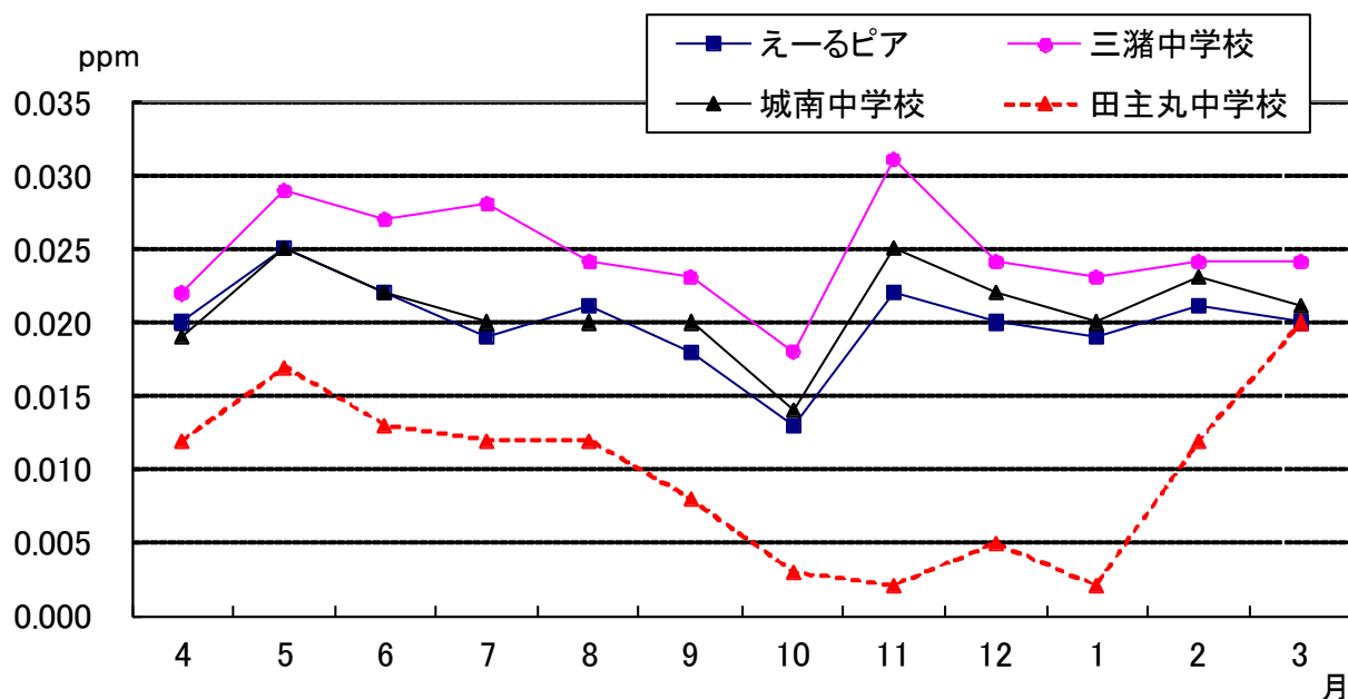
図2-1-8 平成29年度 浮遊粒子状物質 年間変化
