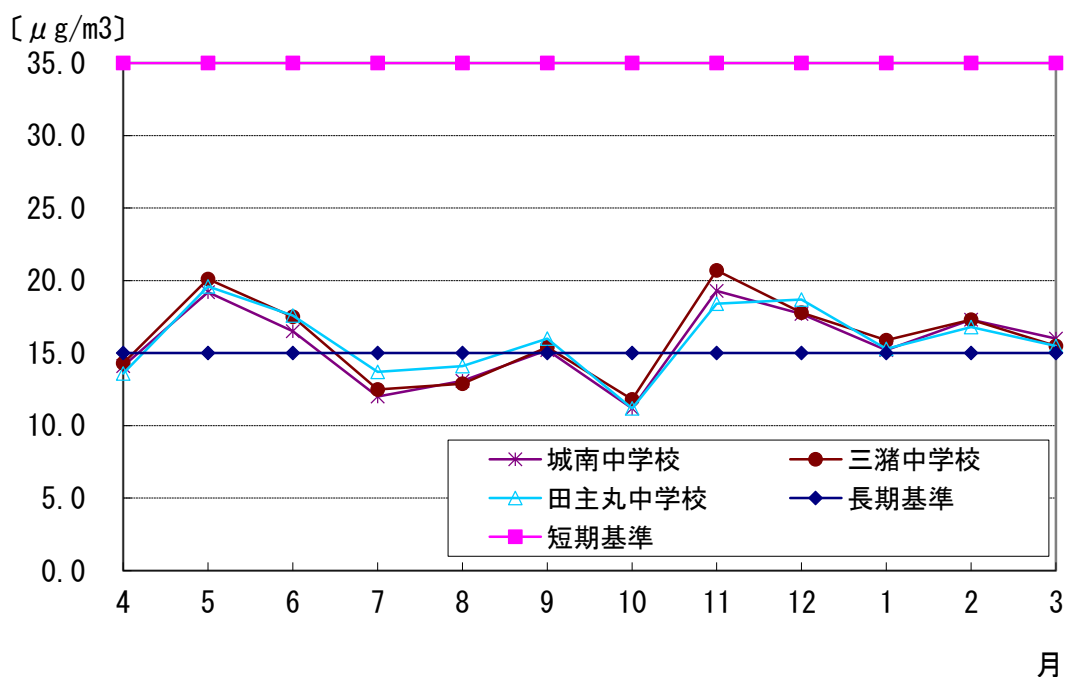
図2-1-10 平成29年度 PM2.5濃度 年間変化(月平均値)
