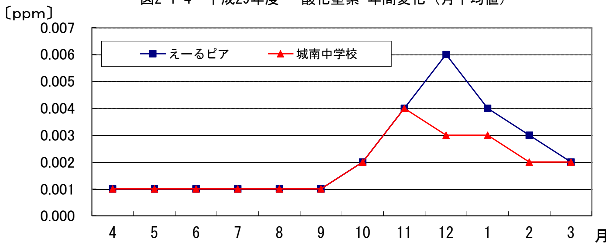
図2-1-4 平成29年度 一酸化窒素 年間変化（月平均値）
