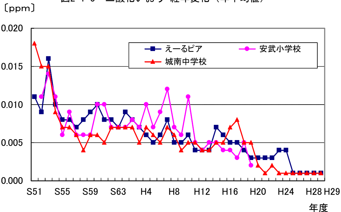
図2-1-3 二酸化いおう 経年変化(年平均値)
