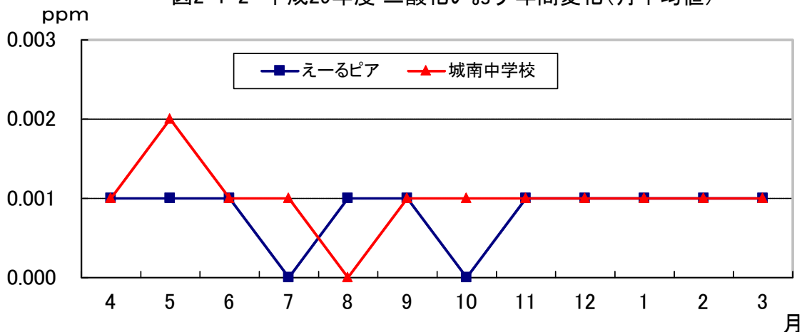
図2-1-2 平成29年度 二酸化いおう 年間変化(月平均値)
