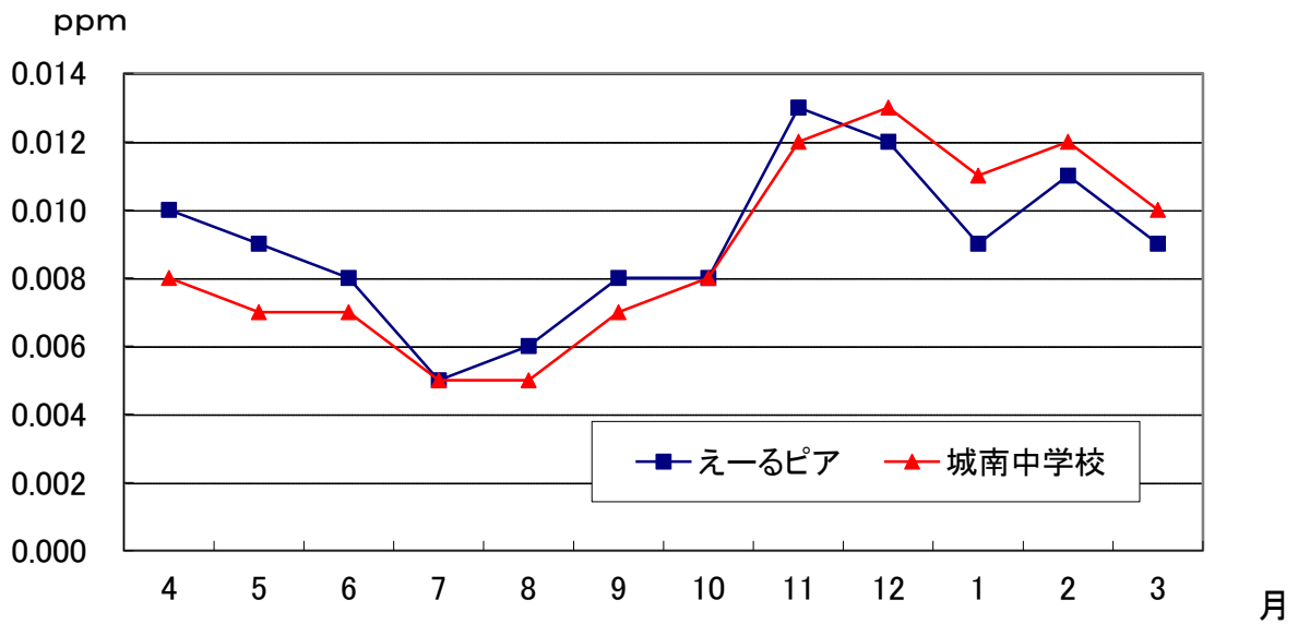
図2-1-6 平成29年度 二酸化窒素 年間変化(月平均値)
