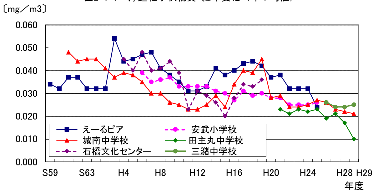
図2-1-9 浮遊粒子状物質 経年変化（年平均値）
