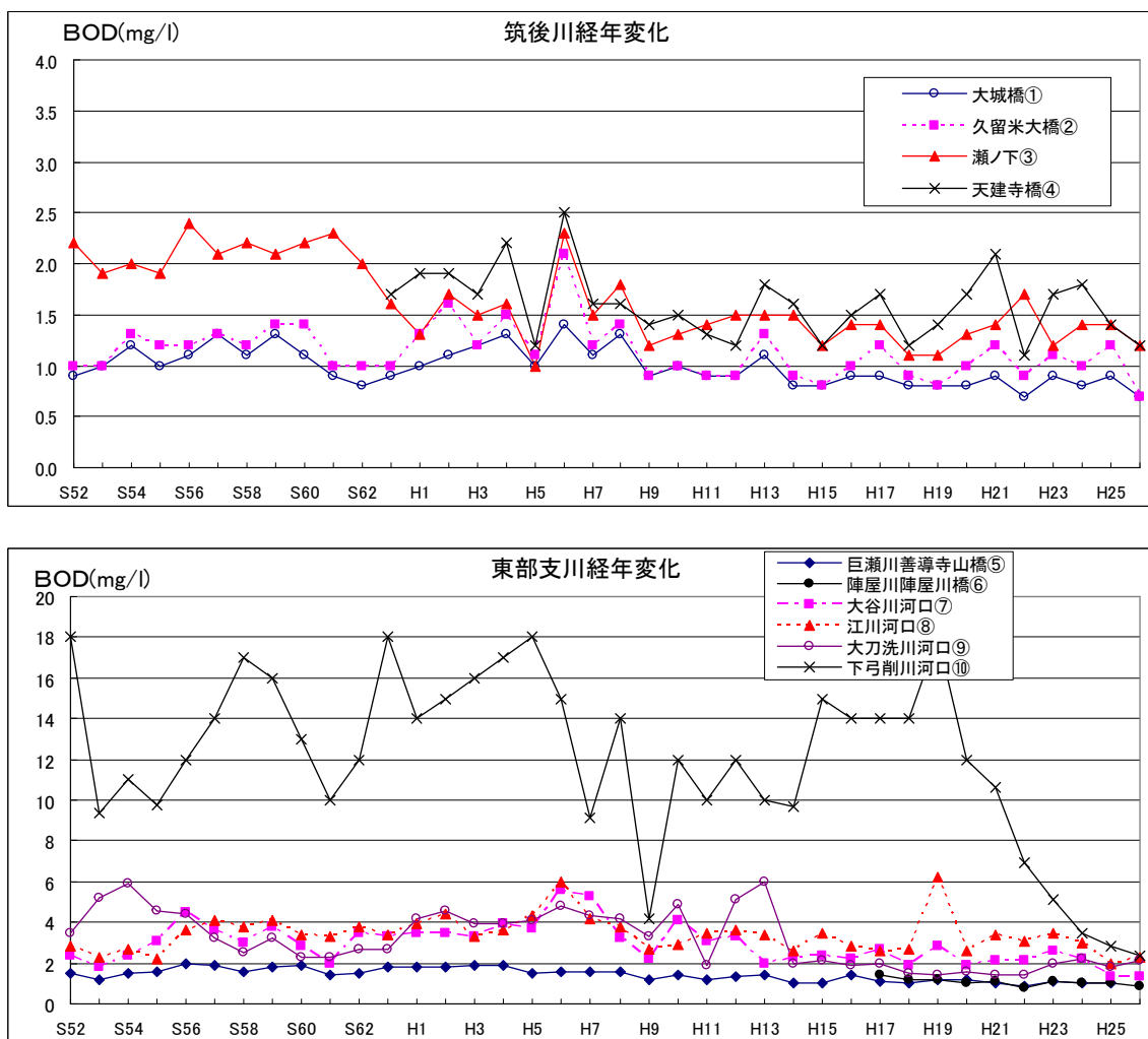
図2-2-3 主要河川水質経年変化
