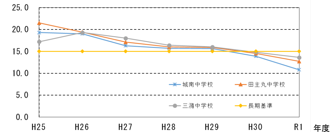
図2-1-11 PM2.5濃度経年変化
