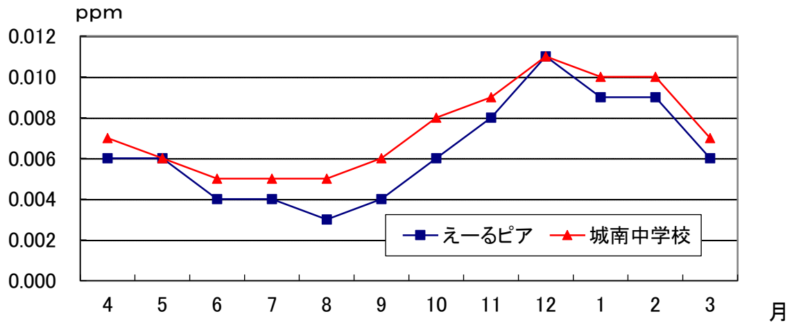
図2-1-6 令和元年度 二酸化窒素 年間変化(月平均値)
