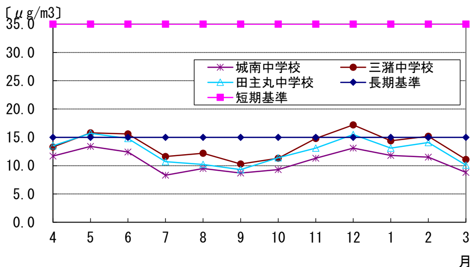
図2-1-10 令和元年度 PM2.5濃度 年間変化(月平均値)
