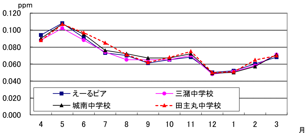
図2-1-18 令和元年度 光化学オキシダント年間変化 （昼間の1時間値の最高値）
