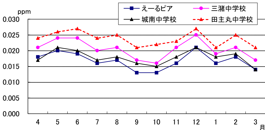
図2-1-8 令和元年度 浮遊粒子状物質 年間変化
