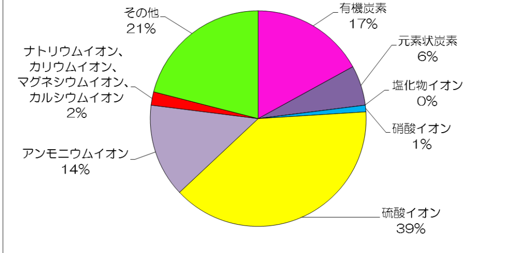
図 2-1-14 平成 29 年度 PM2.5 成分測定結果
