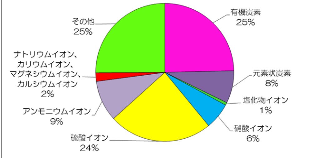
図 2-1-15 平成 28 年度 PM2.5 成分測定結果
