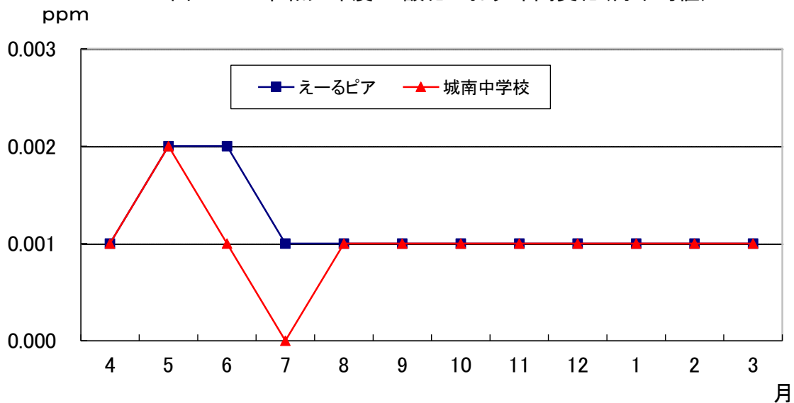
図2-1-2 令和元年度 二酸化いおう 年間変化(月平均値)
