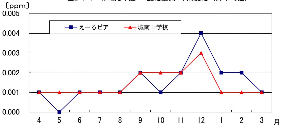
図2-1-4 令和元年度 一酸化窒素 年間変化（月平均値）
